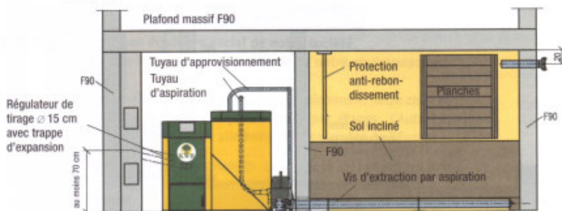
Élévation
